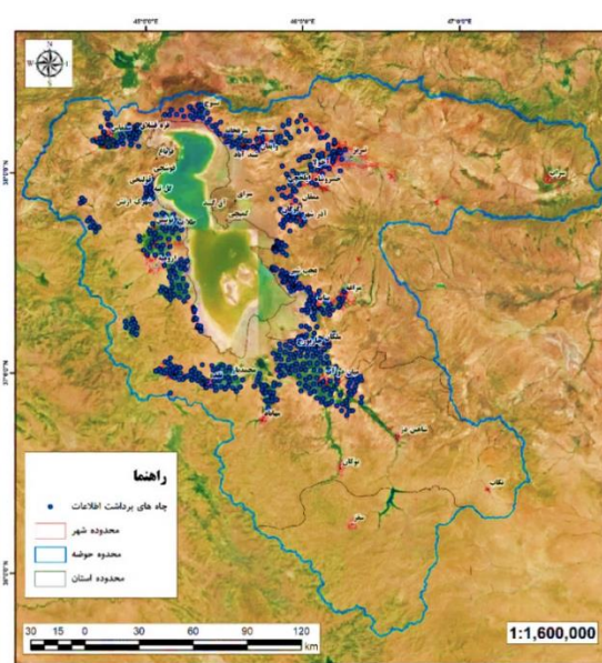
شکل ۲. موقعیت چاه‌های مورد استفاده
