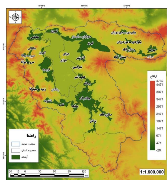
شکل ۳. آبخوان‌های حوزه آبریز دریاچه ارومیه
