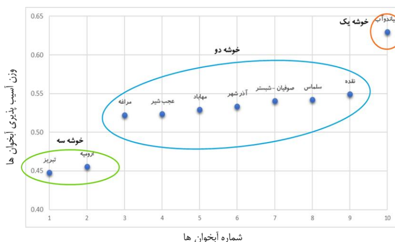
شکل ۲۱. خوشه‌بندی اوزان آبخوان‌ها بر اساس روش K-Mean
