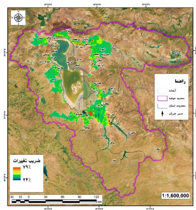
شکل ۵. ضریب تغییرات در محدوده مورد مطالعه
